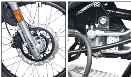
(1) Sensor de velocidad de la rueda (2) Unidad de control electrónico hidráulico (HECU)
