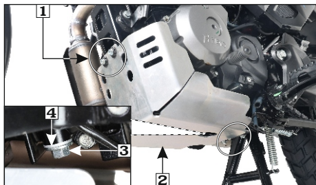
(1) Pernos de la placa de protección (2) Placa de protección (3) Perno de drenaje (4) Arandela selladora
